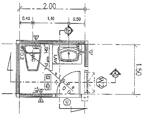
แปลนห้องน้ำ-1 1:50
