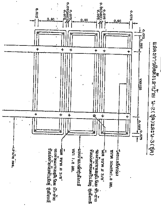
แบบสถาปัตย์โครงสร้างป้าย น-2 (ชุด) และ น-3 (ชุด)
