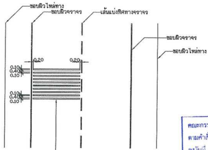
แบบขยาย RUMBLE STRIPS สีทอง โพลีเอสเตอร์ หนา 5.00 มม. สีขาว จำนวน 10 แถบ
