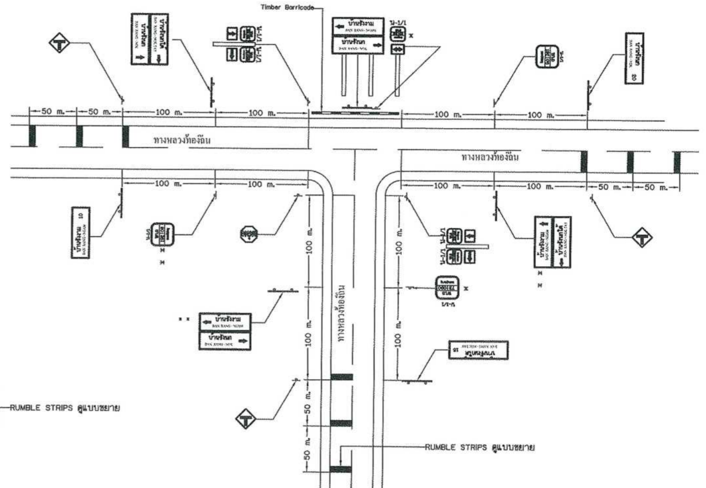
แสดงการติดตั้งป้ายจราจรบริเวณสามแยก ( เชื่อมทางหลวงท่งถิ่น )
