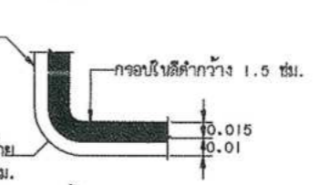
แสดงมุมป้ายแนะนำนอกทิศทาง ( น-6 ถึง น-19 )
