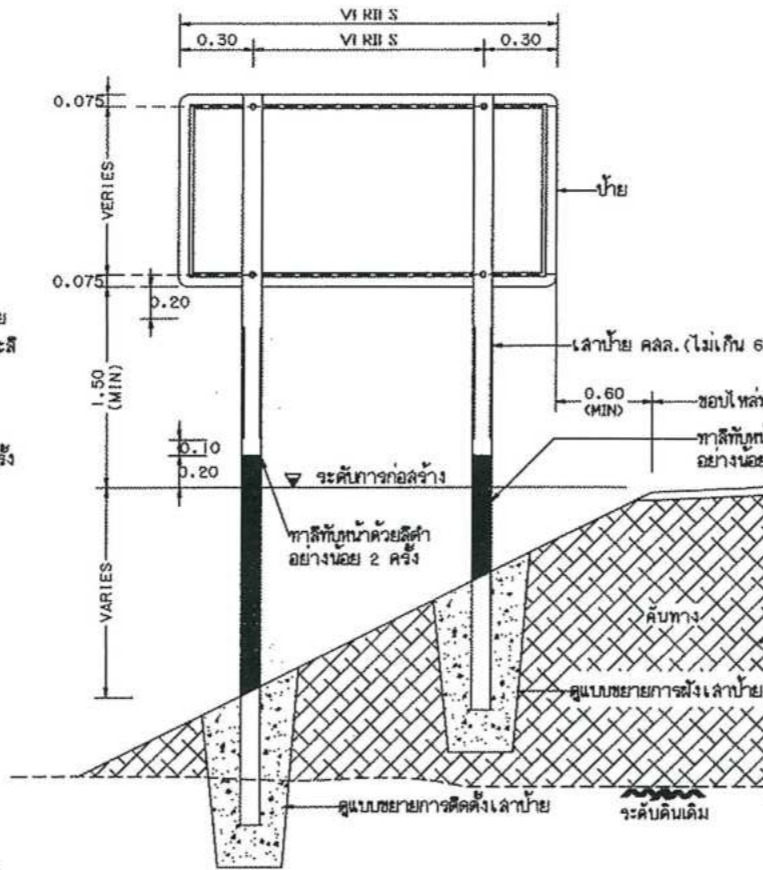
แปลนการปักเสาป้ายแนะนำ น-2 น-3 และ น-5
