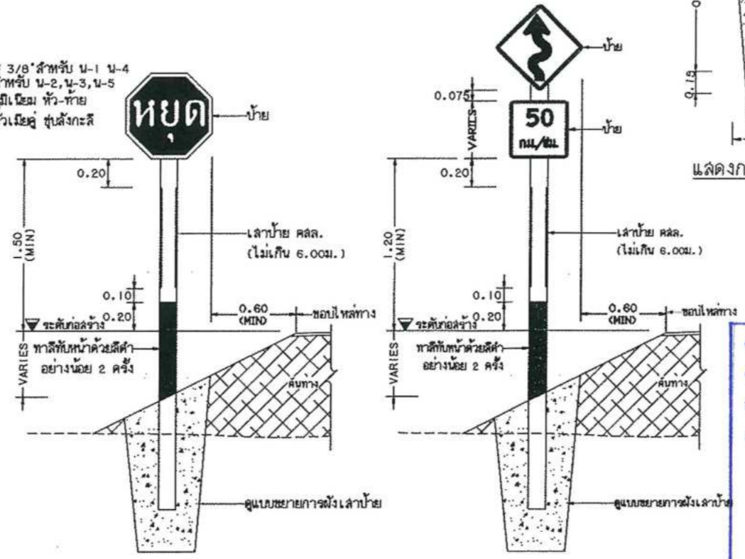
แปลนการปักเสาป้ายบังคับและป้ายเตือน
