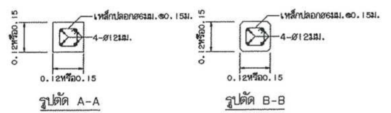
รูปลัด เสาป้าย
