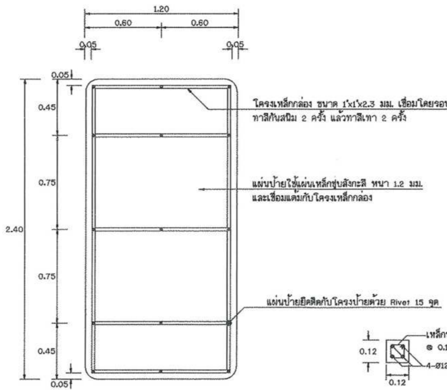
แสดงด้านหลังป้ายกำหนดน้ำหนักรถทุก
