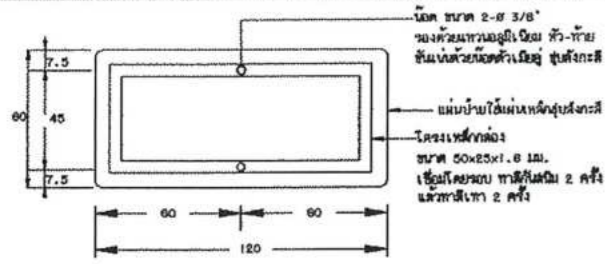
แปลนการยึดโครงป้ายโครงการ น-1
