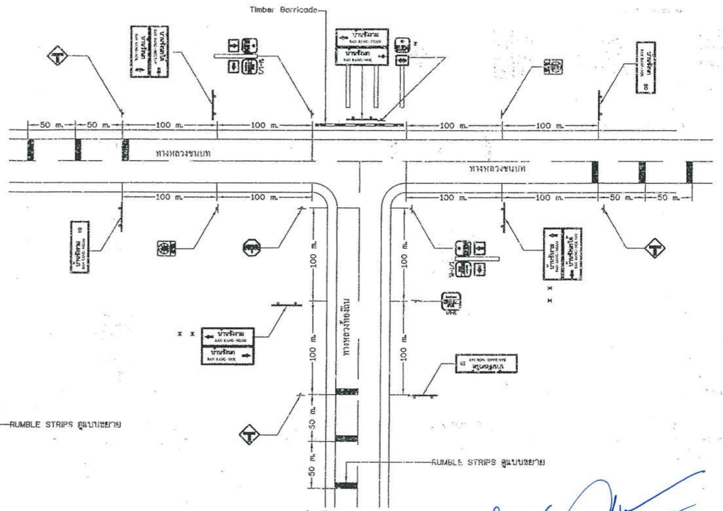
แสดงการติดตั้งป้ายจราจรบริเวณสามแยก ( เชื่อมทางหลวงชนบท ) แบบคู่มือประกอบกาหนดครุฑากถน
