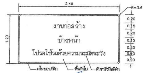
ป้ายเตือนการก่อสร้าง
