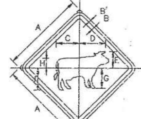
เว้นขอบป้าย สีเหลืองสะท้อนแสง เส้นขอบป้าย สีดำไม่สะท้อนแสง พื้นป้าย สีเหลืองสะท้อนแสง เครื่องหมาย สีดำไม่สะท้อนแสง
