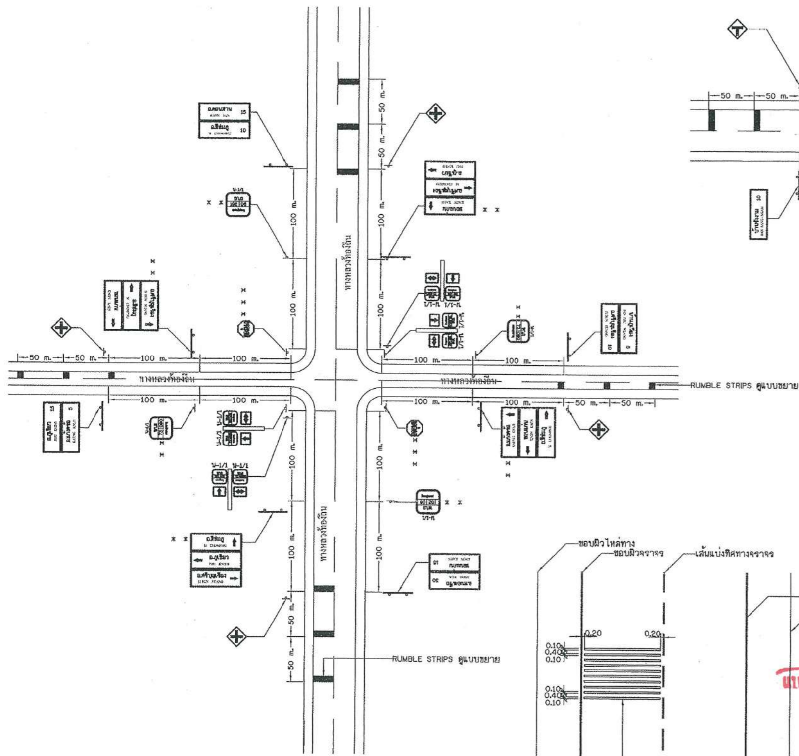
แสดงการติดตั้งป้ายจราจรบริเวณแยก ( เชื่อมทางหลวงท้องถิ่น )
