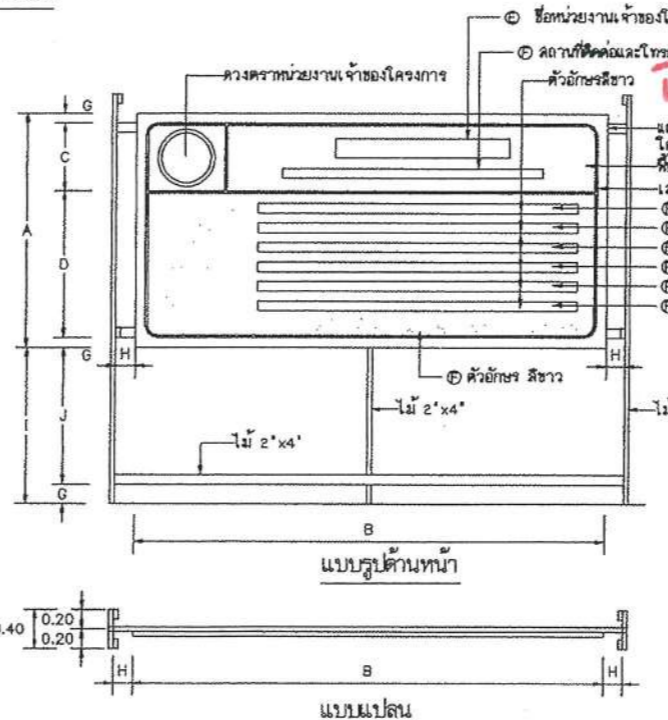
แปลนป้ายรายละเอียดงานก่อสร้าง
