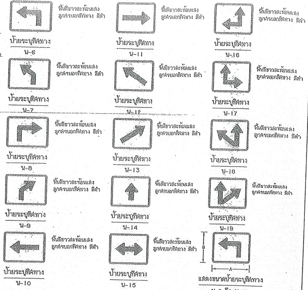
แสดงขนาดป้ายระบุทิศทาง น-6 ถึง น-19
