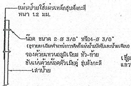
แสดงการติดตั้งป้ายบังคับ,ป้ายเตือน
