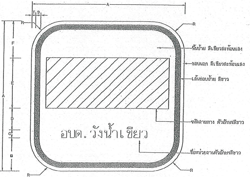
ป้ายหมายเลขทางหลวงท้องถิ่น น-1/1 (กรณีติดตั้งป้ายในเขตทางของทางหลวงและทางหลวงชนบท)
