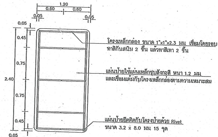
แสดงการยึดแผ่นป้ายกับโครงเหล็ก
