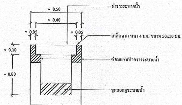
รูปตัดรางระบายน้ำ
