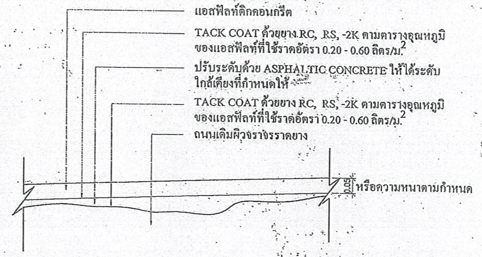
รายละเอียดงาน OVERLAY ASPHALTIC CONCRETE
