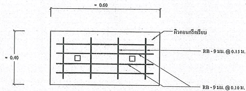
แบบขยายฝารางระบายน้ำ
