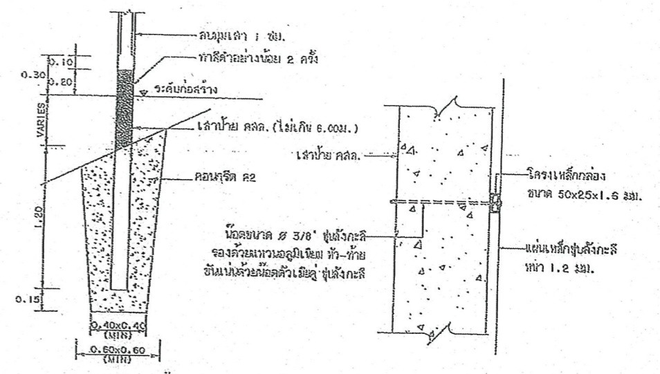
แสดงการส่งเสาป้าย
