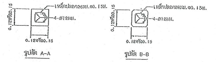
รูปตัดเสาป้าย (ดูขยายเขต ข้อ 4)
