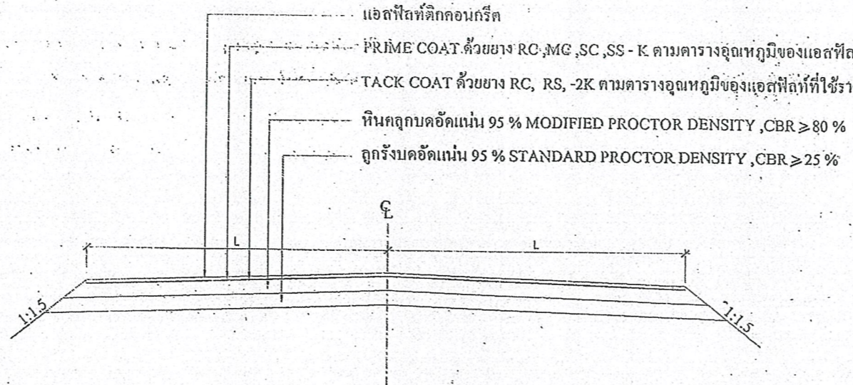
รูปตัดถนน แอสฟัลท์ติก คอนกรีต
