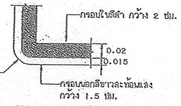
แสดงมุมป้ายหน้า (น-2 ถึง น-5)
