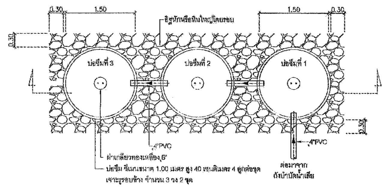
แปลนปอซีม
