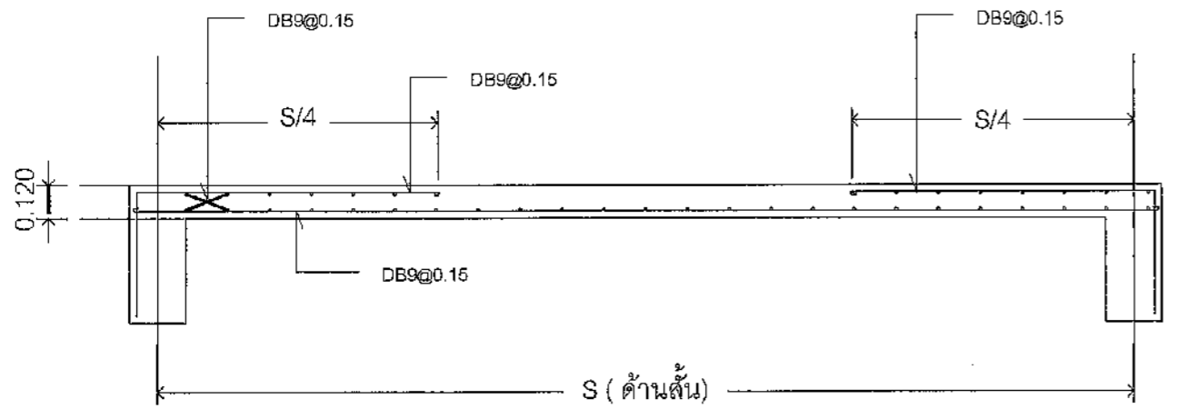
พื้น S2
