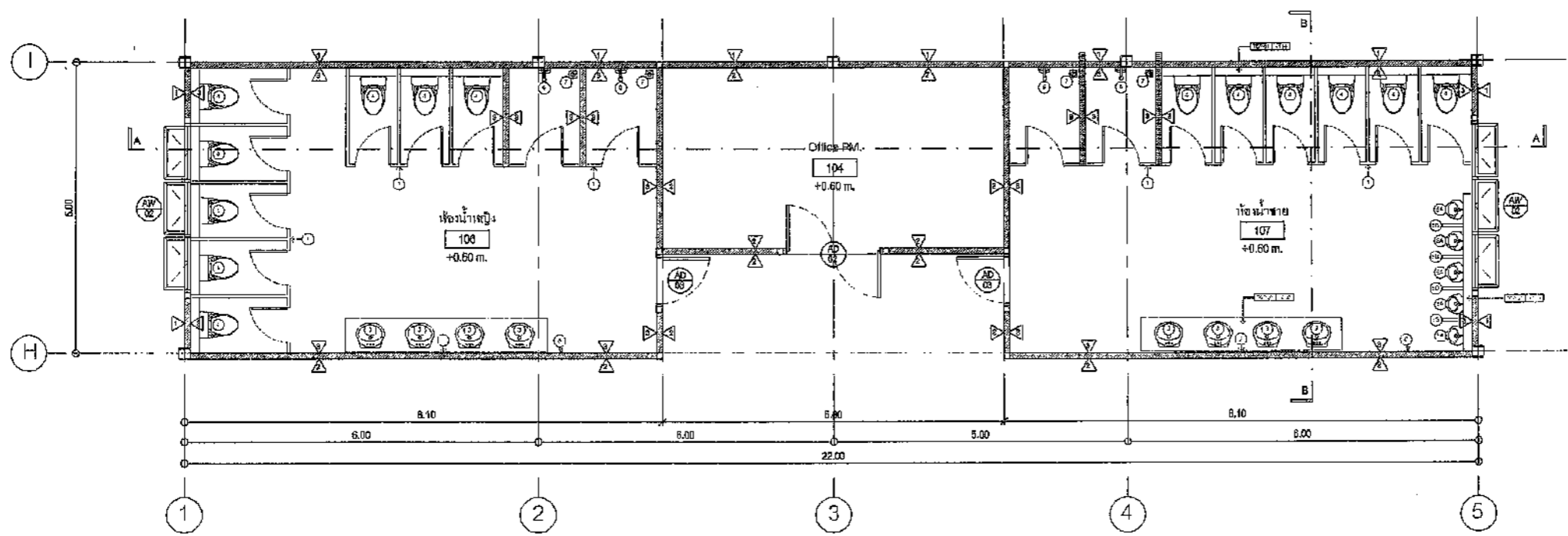
แบบขยายห้องน้ำ เฝ้งพื้น SCALE 1:100 A3
