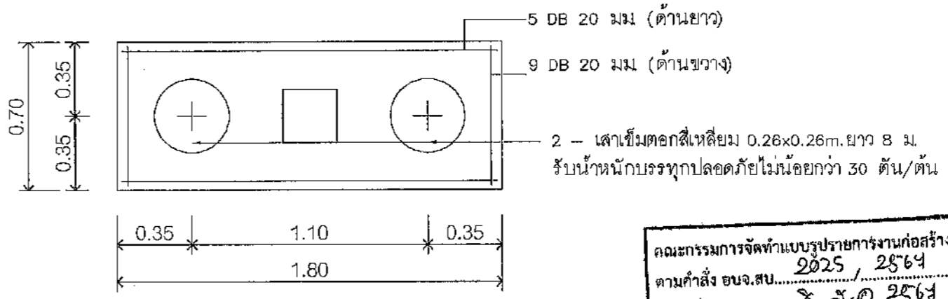
F2 แบบขยายฐานราก, ตอม่อ, เส้า SCALE 1:25
