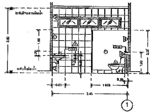
แบบขยายห้องน้ำ : รูปตัด B SCALE 1:100 A3
