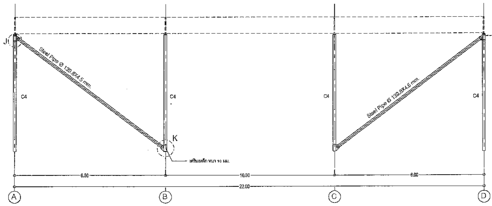
แบบขยาย FRONT STEEL PIPE SCALE 1:125 A3
