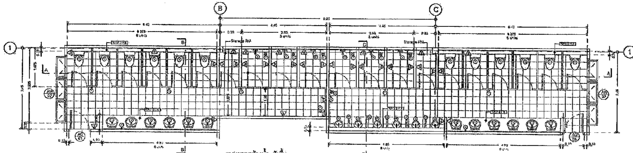
แบบขยายห้องน้ำ : ค้างทิ้ง SCALE 1:100 A3
