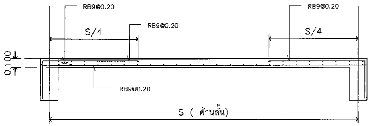
พื้น S1 SCALE 1:25 A3
