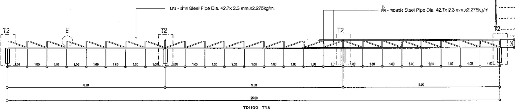
TRUSS T3A SCALE 1:100 A3
