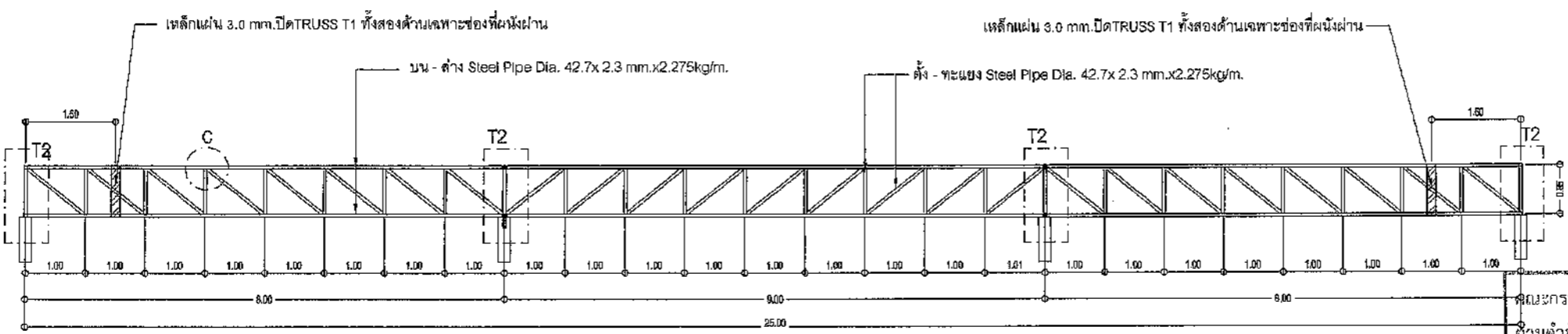
TRUSS T3 SCALE 1:100 A3
