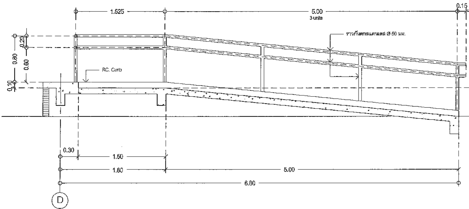
แบบขยายจุกบันได ST-01
