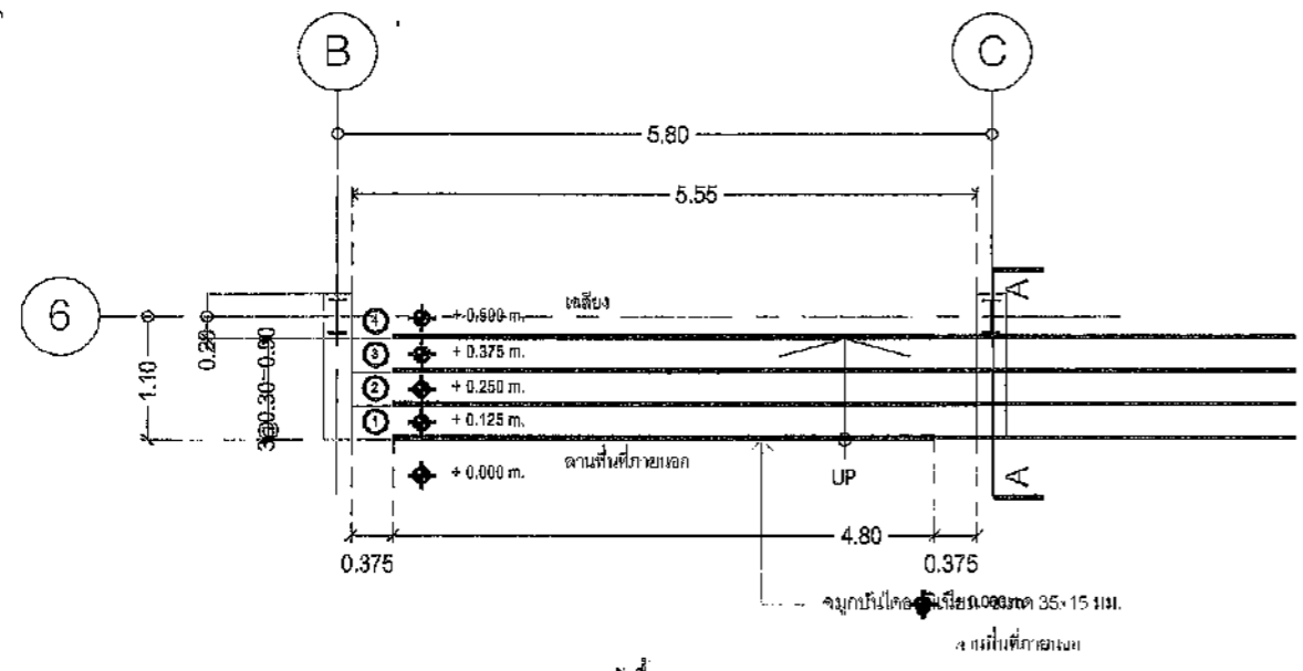
แบบขยาย ST-01, R-01 : กิ่งพื้น SCALE 1:75 A3
