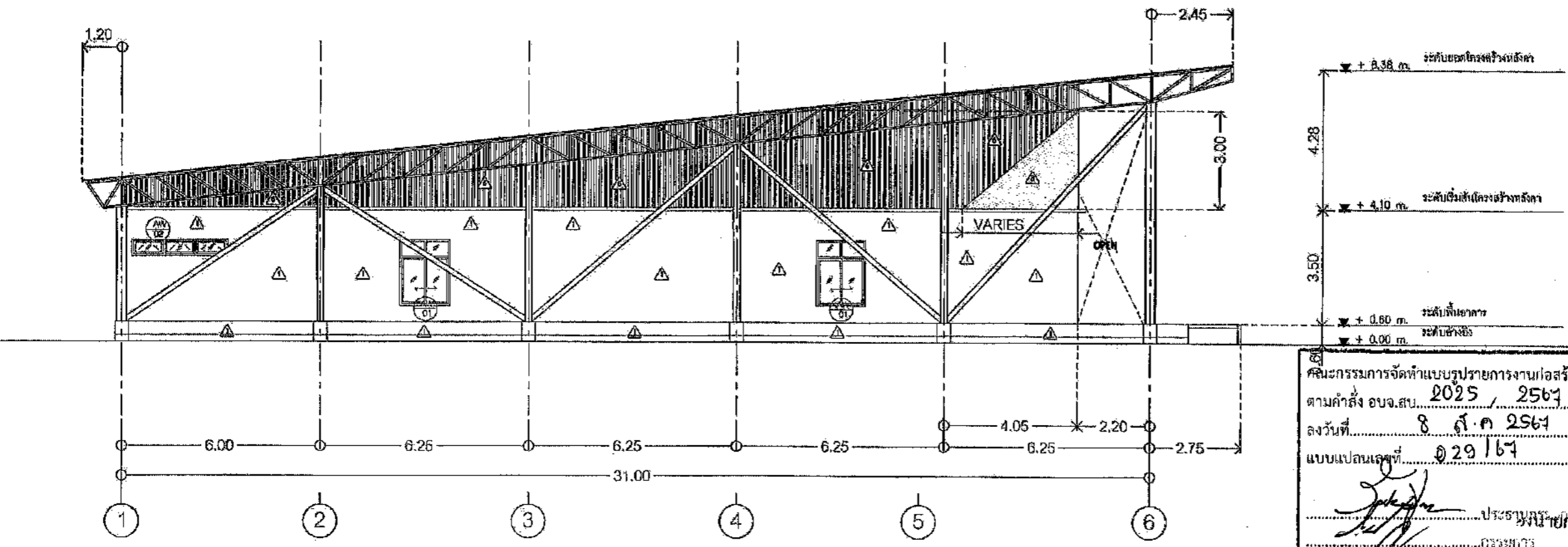
รูปด้าน 2 SCALE 1:150 A3
