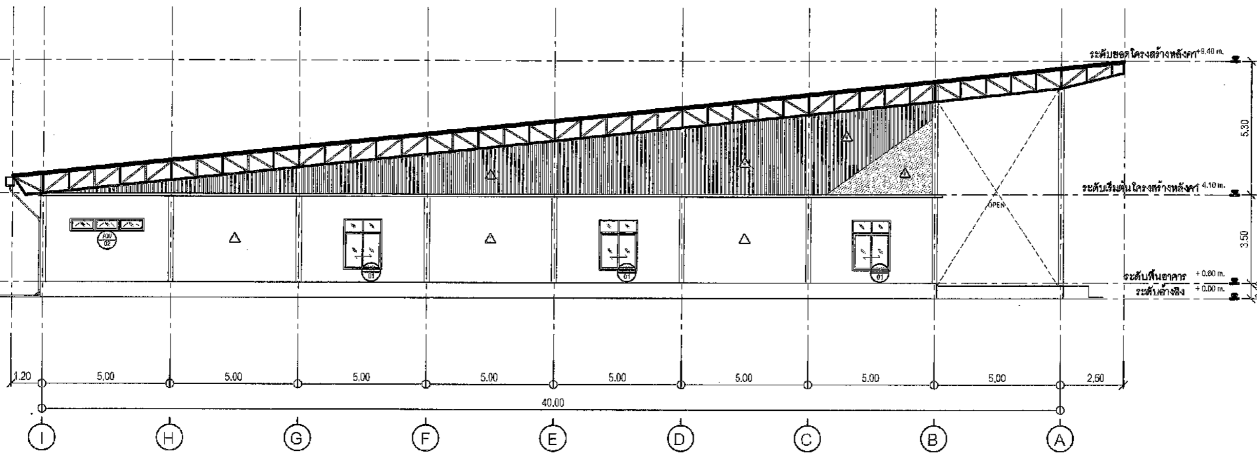
รูปด้าน 3 SCALE 1:150 A3
