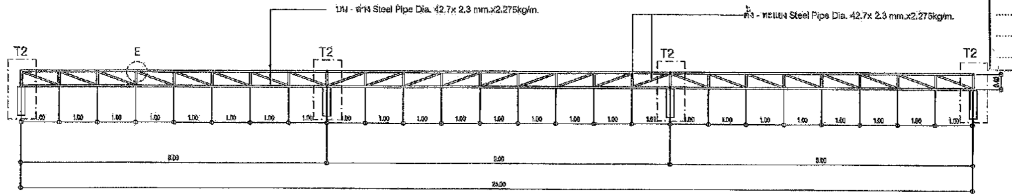
TRUSS T3A SCALE 1:100 A3
