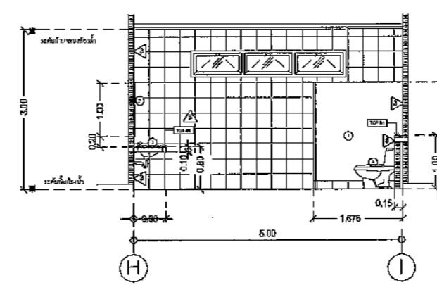
แบบขยายห้องน้ำ รูปตัด B SCALE 1:100 A3
