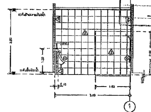
แบบขยายห้องน้ำ : รูปตัด C SCALE 1:100 A3
