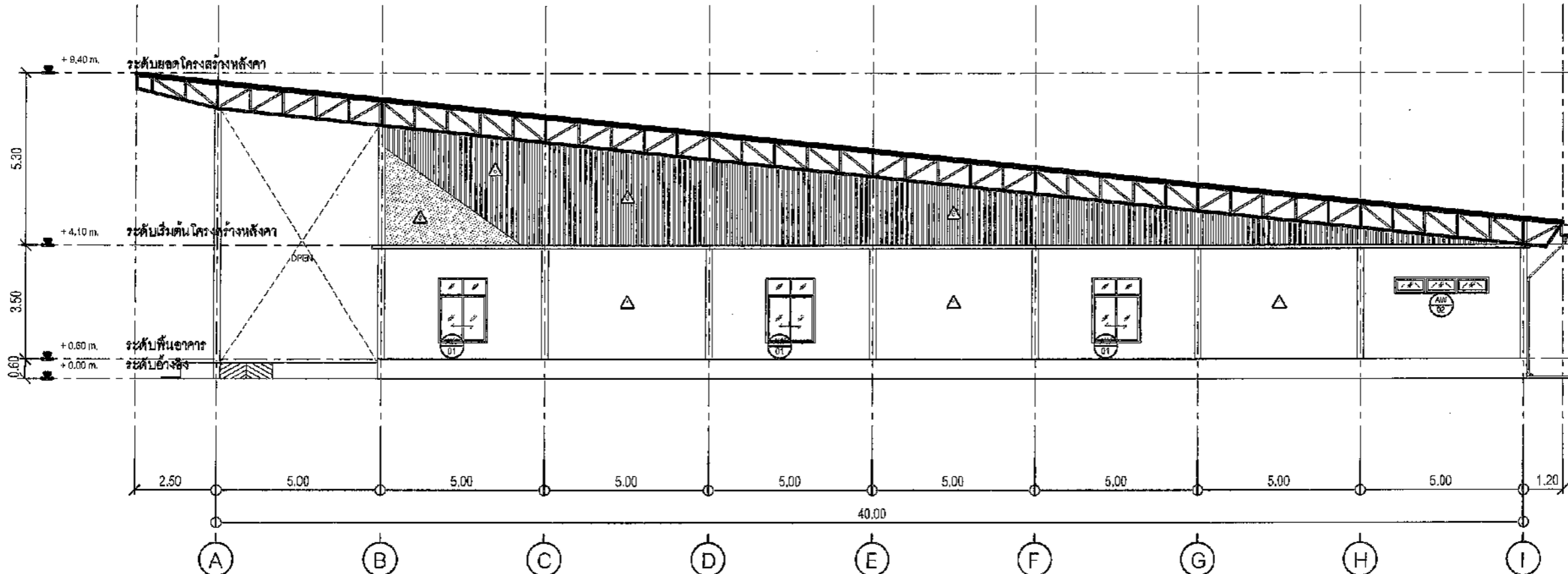
รูปด้าน 1 SCALE 1:150 A3
