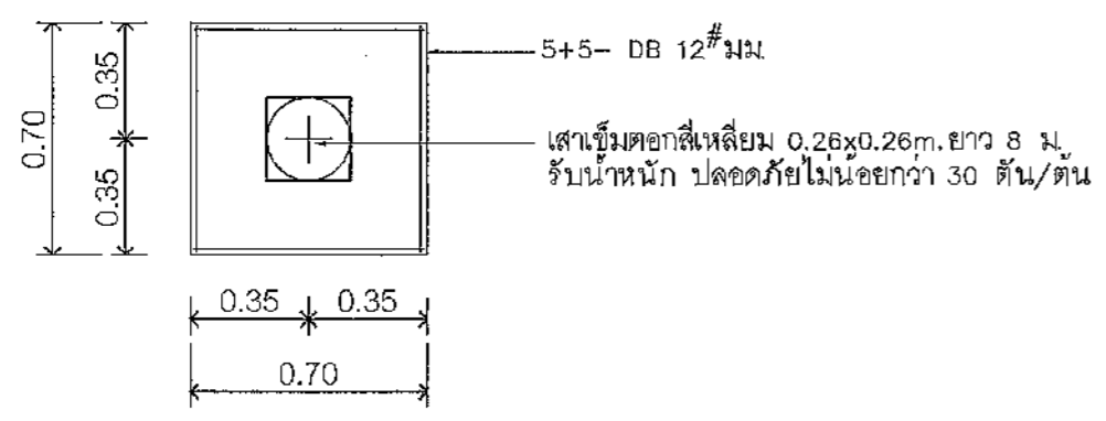
F1 แบบขยายฐานราก, ตอม่อ, เส้า SCALE 1:25
