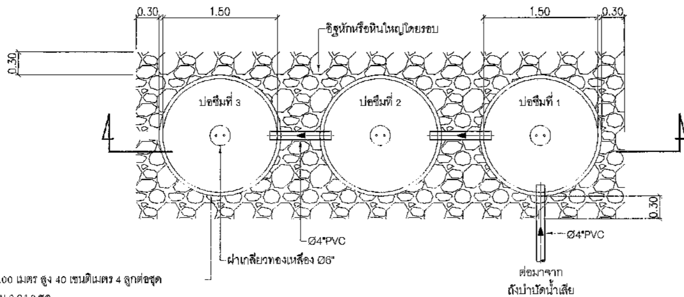
แปลนบ่อซีเมนต์
