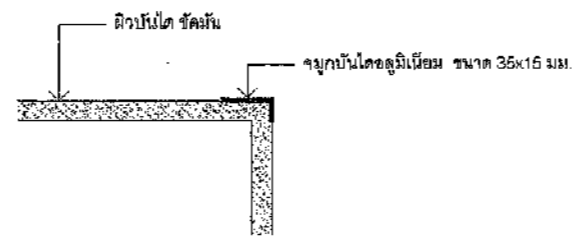
แบบขยายจุกบันได ST-01
