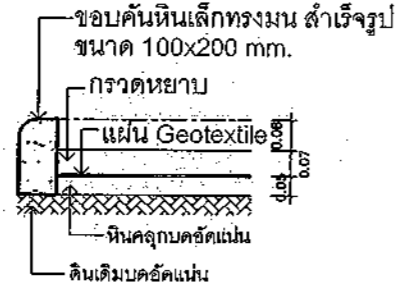
แบบขยาย - 01 : สันนามเปิดช่อง
