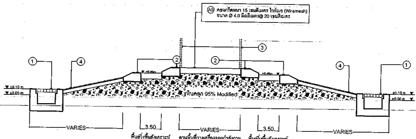
รูปตัด A
