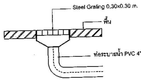
แบบขยาย Floor Drain
