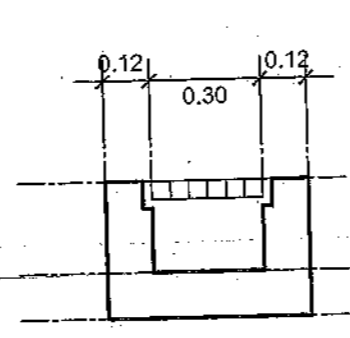
แบบขยาย : RC gutter
