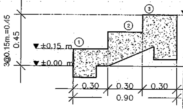
แบบขยายบันได : ST-01
