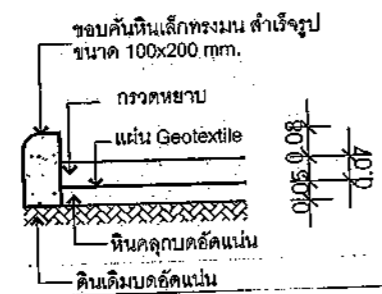
แบบขยาย - 01 : สนามเปิดอง
