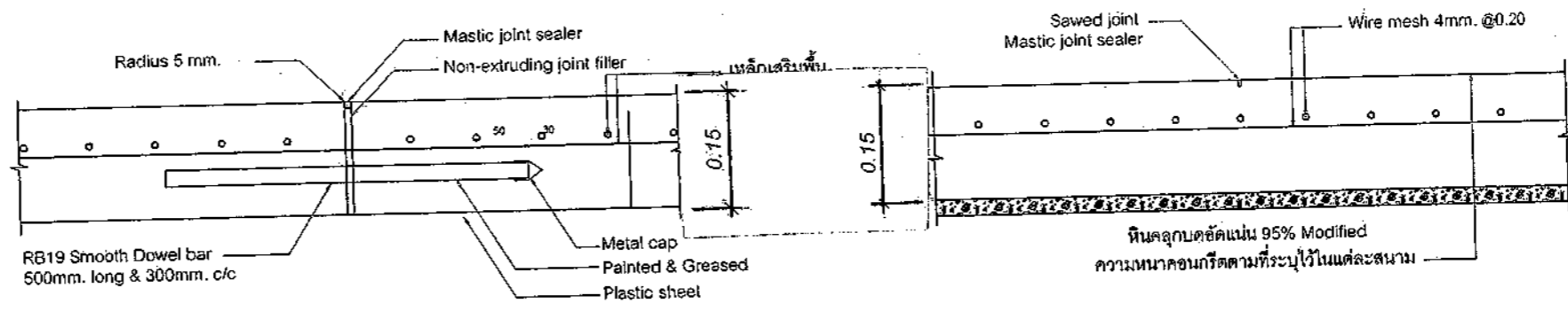
แบบขยายโครงสร้างพื้น : สำหรับพื้นที่ ค.ส.ล. ทัวไป
