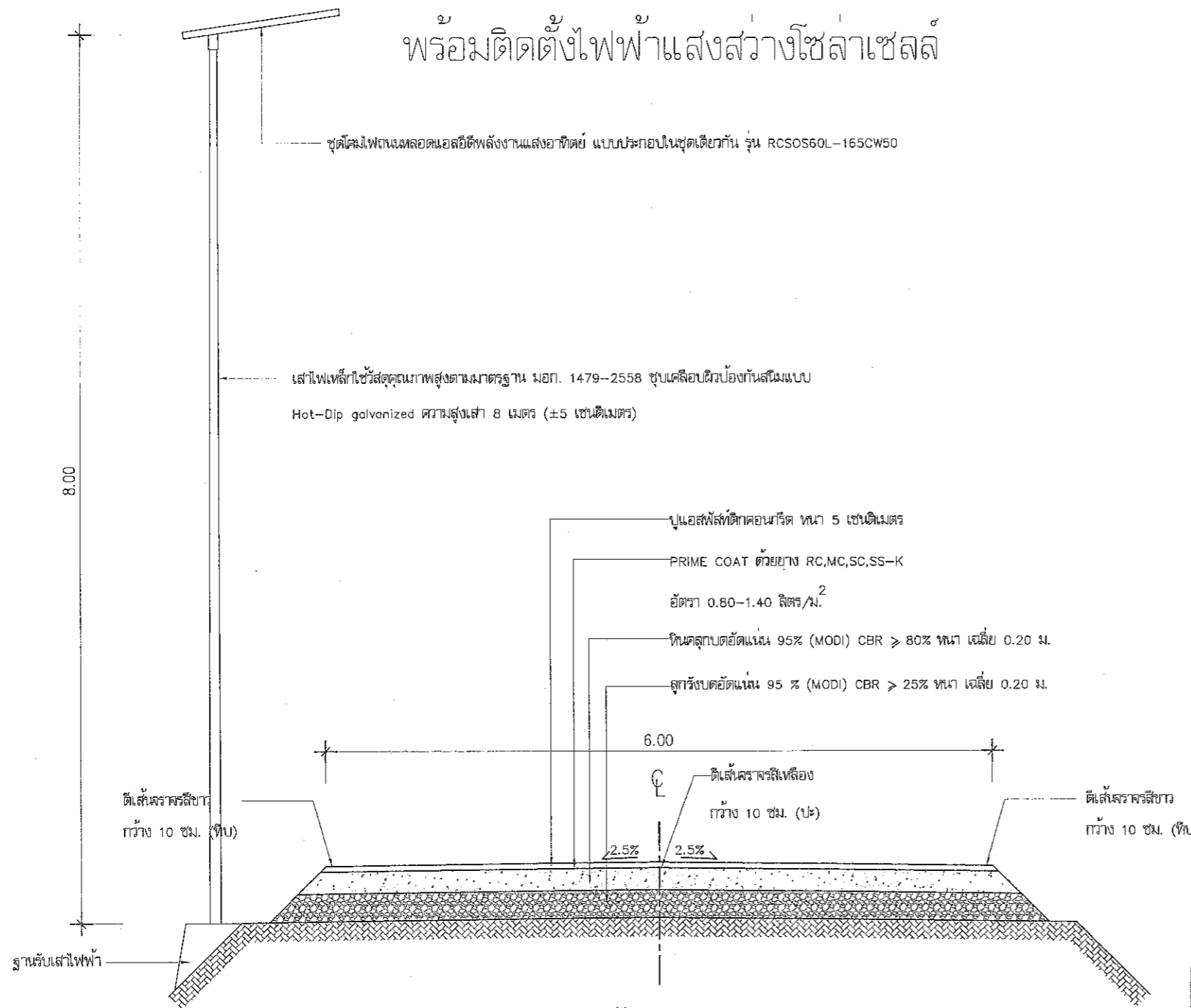
รูปตัดตามขวาง
