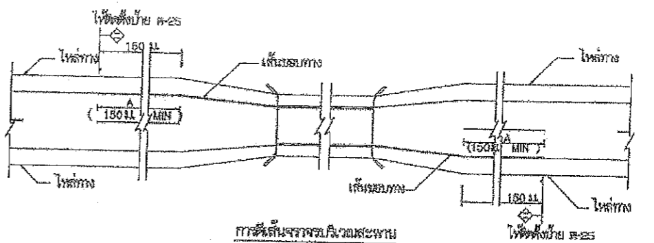
กรณีความกว้างสะพานน้อยกว่าความกว้างผิวจราจรเดิม
