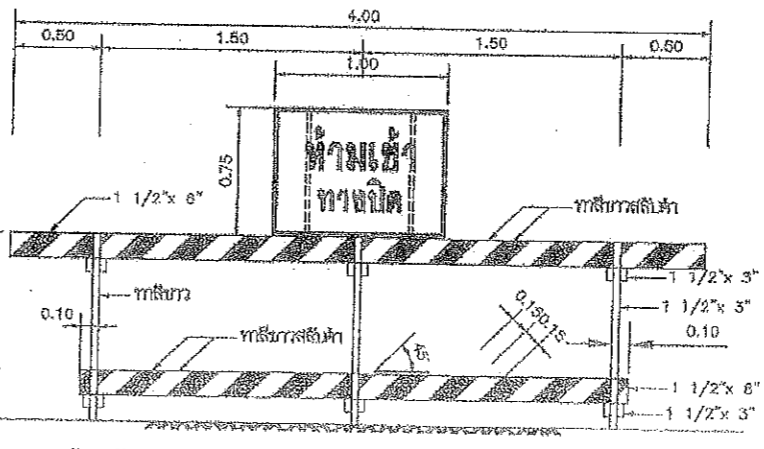
แท่งทึบทำด้วยไม้ และป้ายเครื่องหมายจราจร หมายเลข 4
