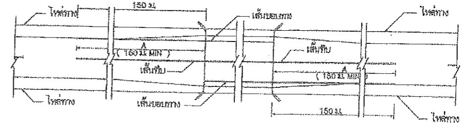
กรณีความกว้างสะพานน้อยกว่าความกว้างผิวจราจรเดิม
