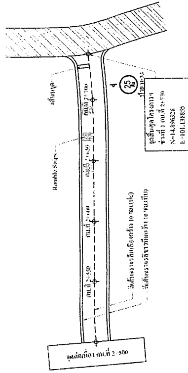
รูปแปลน(ช่วงที่ 1)
