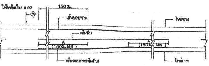
การขึ้นจากรอบ กรณีความกว้างของช่องจราจรลดลง
