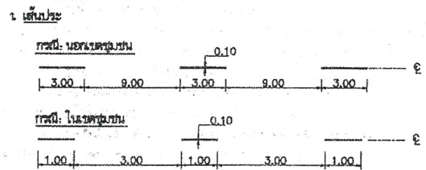
ขนาดและระยะช่องที่หมายจากรอบผิวทาง
