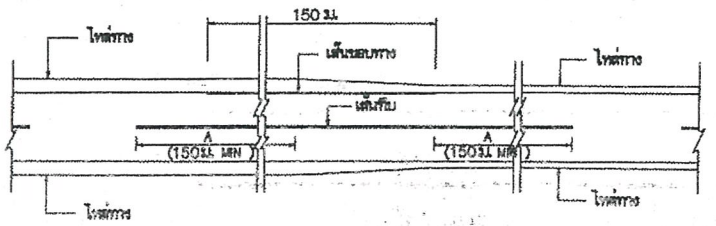
การขึ้นจากรอบ กรณีความกว้างของไหล่ทางลดลง
