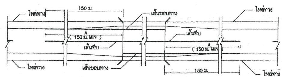
กรณีความกว้างสะพานมากกว่าความกว้างผิวจราจรถนน
