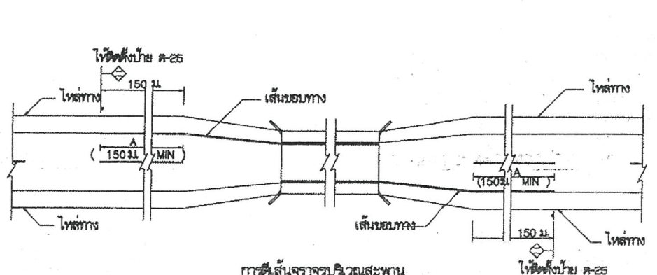
การขึ้นจากรอบบริเวณสะพาน
