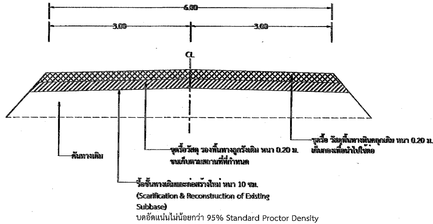
รูปตัด การดำเนินงาน โครงสร้างทางเดิม มาตรฐาน 1:50
