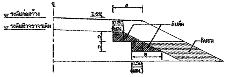
รูปตัดการก่อสร้างลาดคันทางบนถนนเดิม งานตัด ไหล่ (งานตัดเดิม , งานตัดหินหุ , งานตัดหินแข็ง และงานตัดอื่น ๆ)
