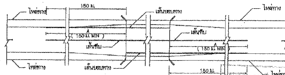
การเส้นความกว้างสะพานน้อยกว่าความกว้างผิวจราจรถนน
