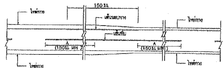
การเส้นจราจร การเส้นความกว้างของไหล่ทางตลอด
