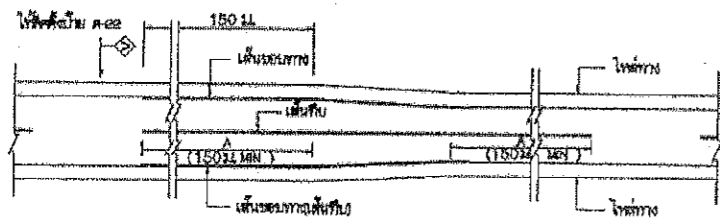
การเส้นจราจร การเส้นความกว้างของช่องจราจรตลอด
