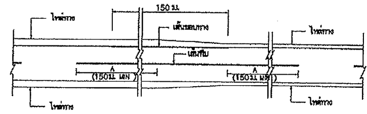
การเส้นจากรอบ กรณีความกว้างของไหล่ทางลดลง
