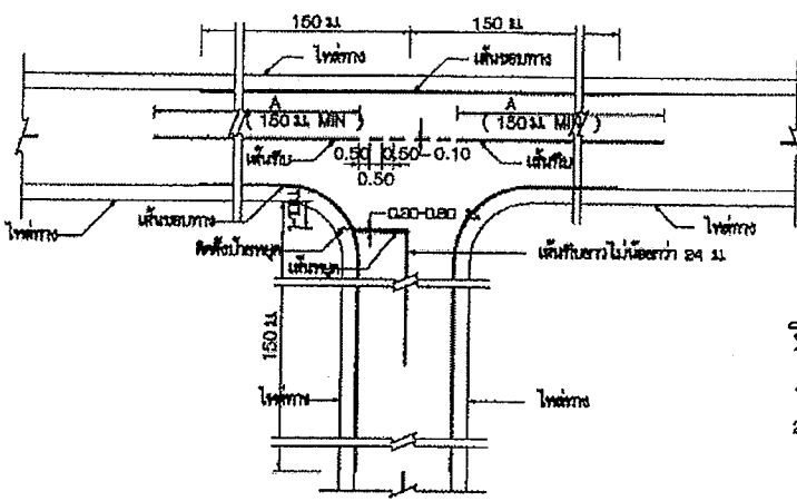
การเส้นจากรอบยก
