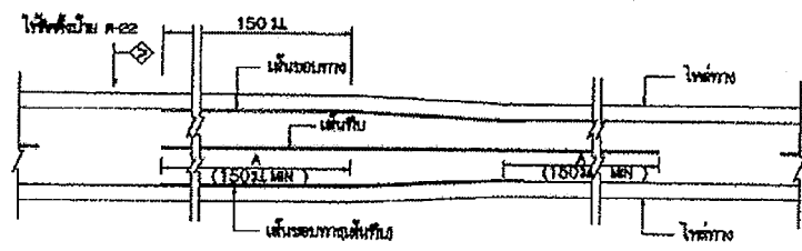
การเส้นจากรอบ กรณีความกว้างของช่องจราจรลดลง
