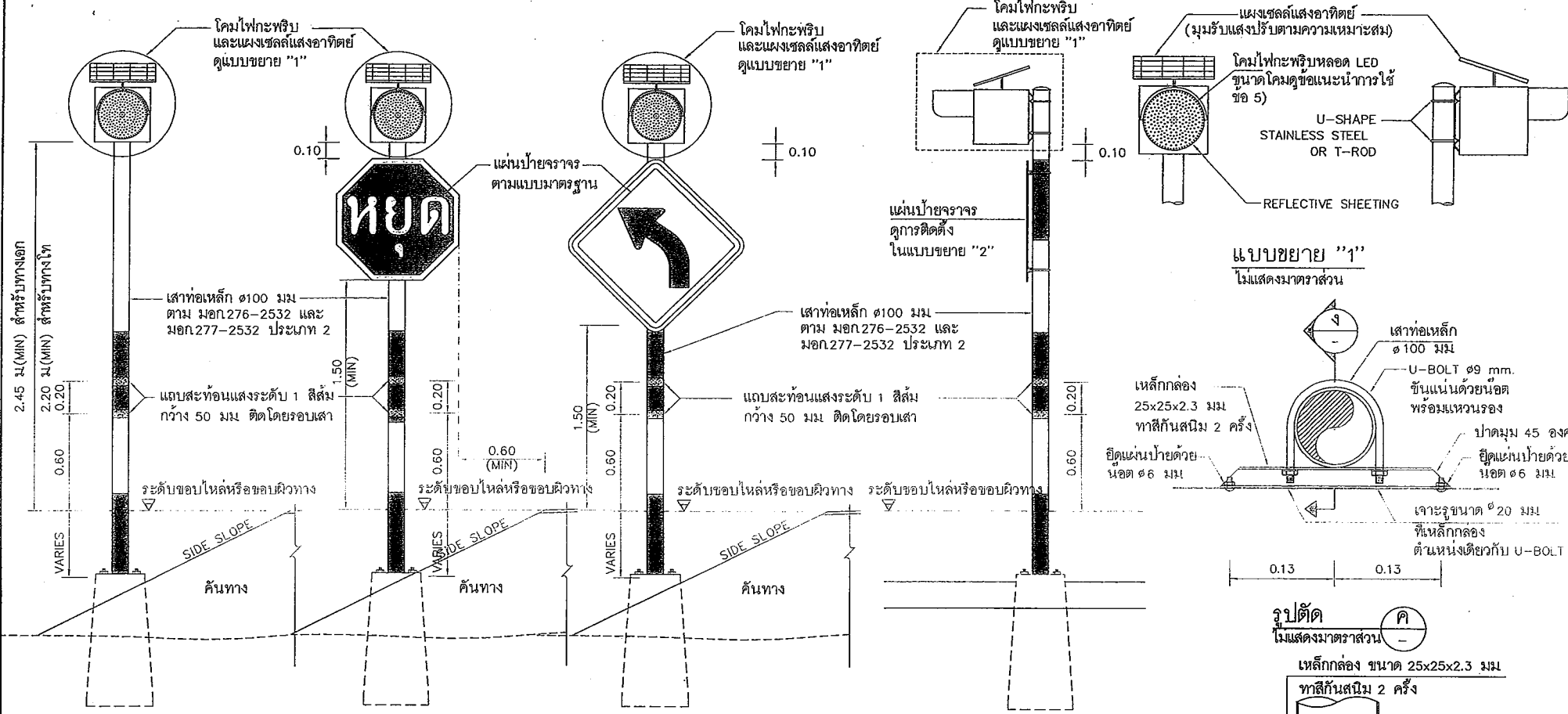
ไฟกะพริบ รูปด้านหน้า ไฟกะพริบร่วมกับป้ายจราจร แสดงการติดตั้งสัญญาณไฟกะพริบอย่างเดียวหรือร่วมกับป้ายบังคับหรือป้ายเตือน (เสาเหล็ก) ไม่แสดงมาตรฐาน
