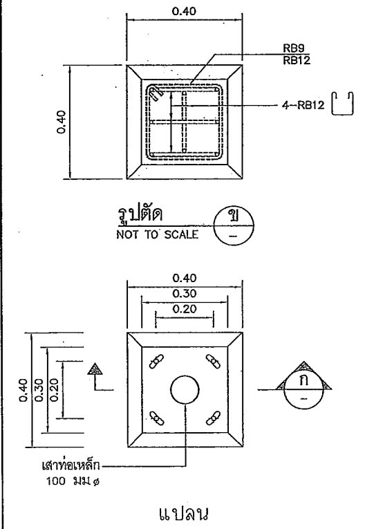
แปลน แบบขยายฐานจาก ไม่แสดงมาตรฐาน
