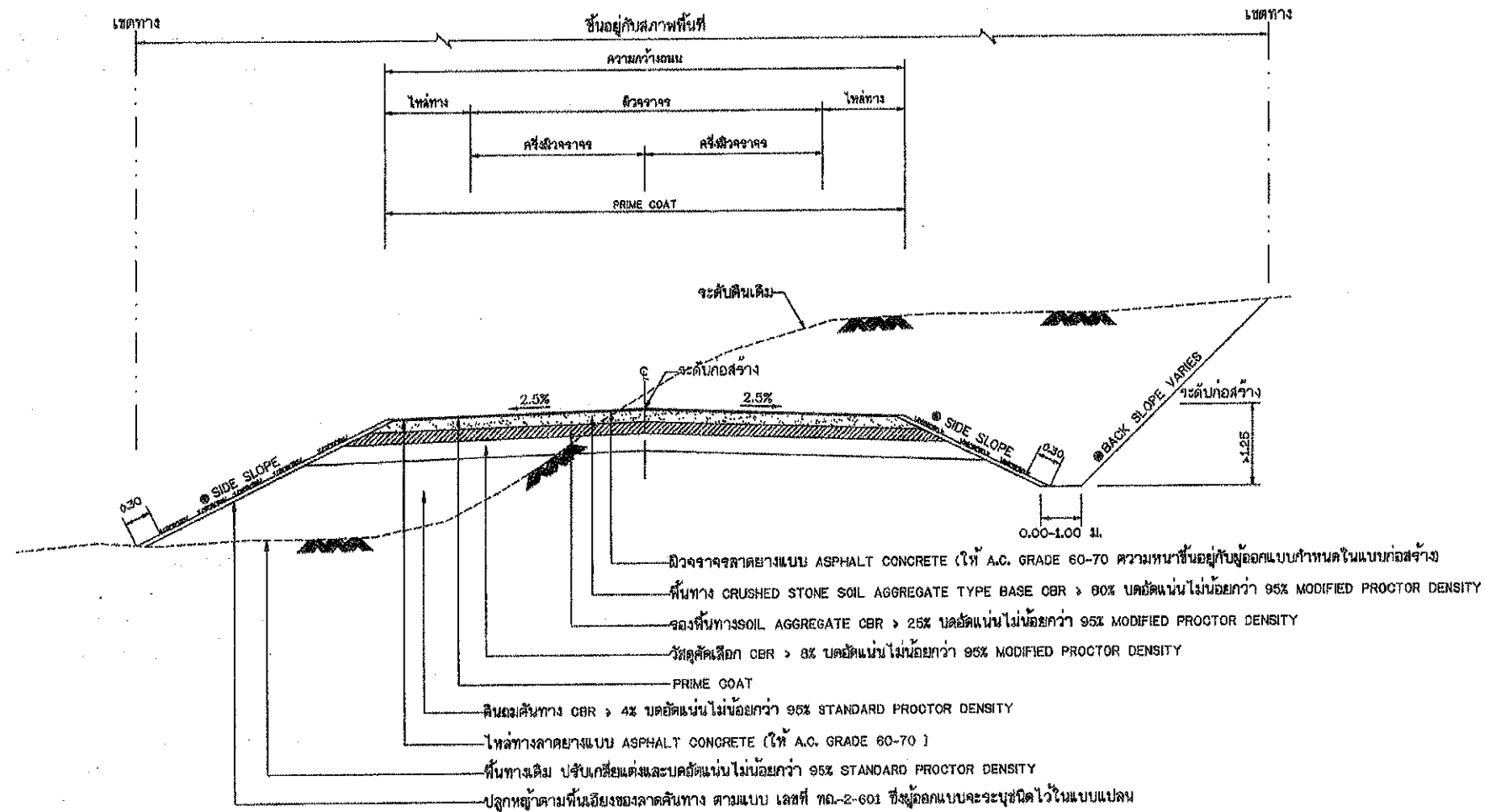
รูปตัดแสดงโครงสร้างถนนดินตัด ดินถมและผสมบิตูวัสดุ
