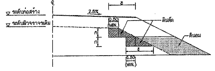
งานตัด ได้แก่ (งานตัดดิน , งานตัดหินหยาบ , งานตัดหินแข็ง และงานตัดอื่น ๆ)
