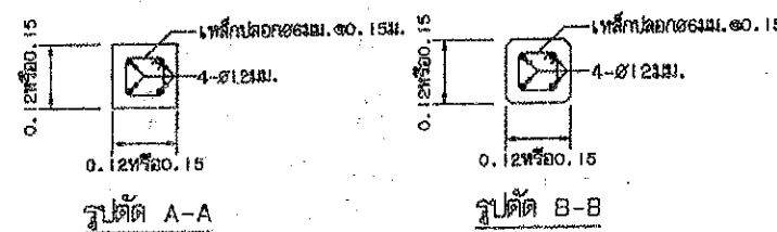
รูปตัดเสาป้าย
