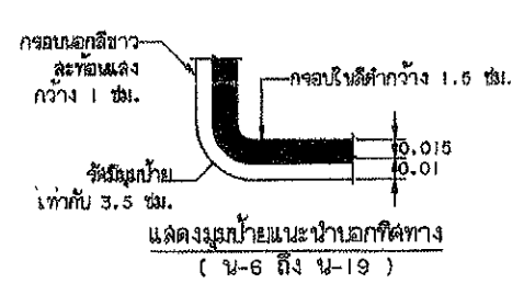
แสดงรูปป้ายแนะนำนอกทิศทาง ( น-6 ถึง น-19 )
