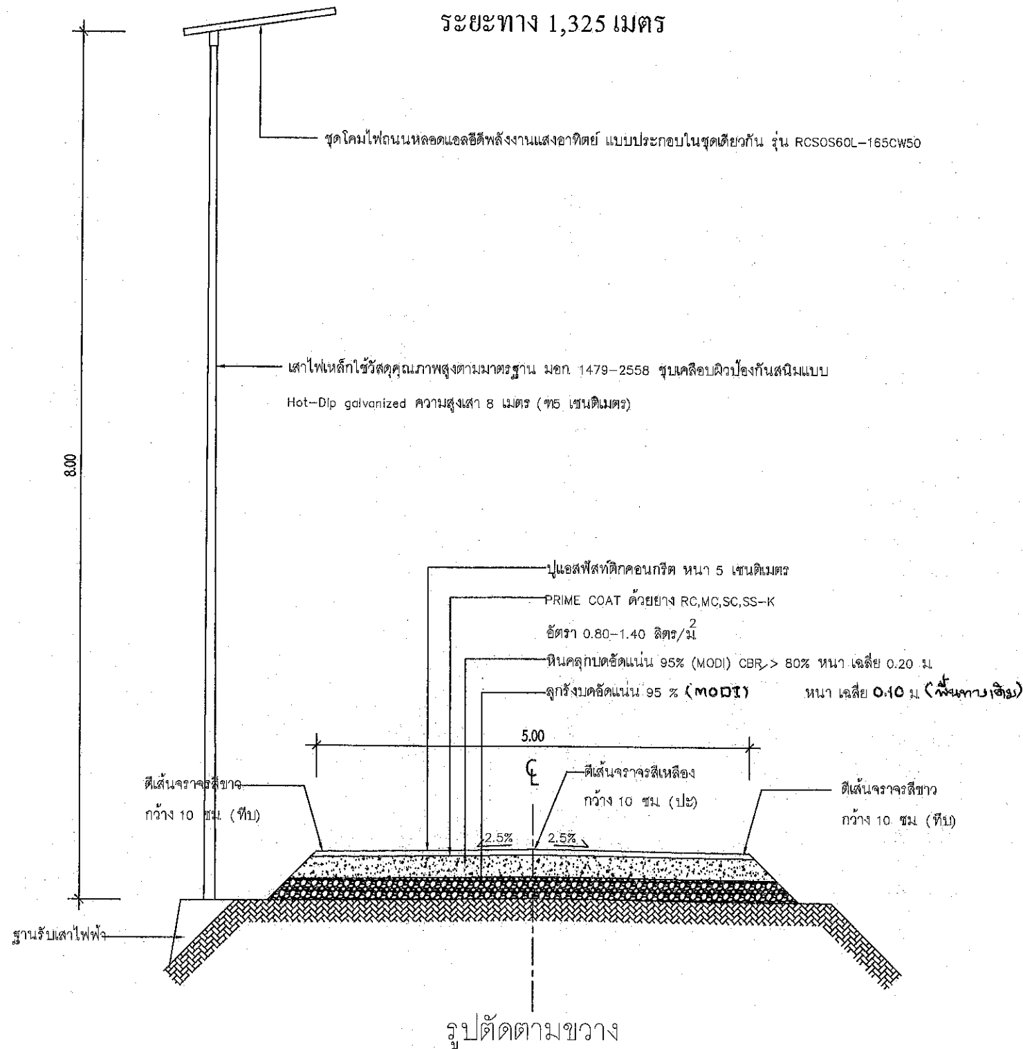
ก่อสร้างถนนลาดยางแบบแอสฟัลต์ติกคอนกรีต (Asphaltic Concrete)
