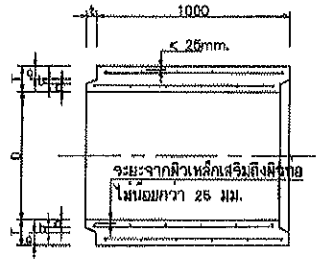
รูปแสดงขนาดแสดงรายละเอียดท่อคอนกรีตเสริมเหล็ก
