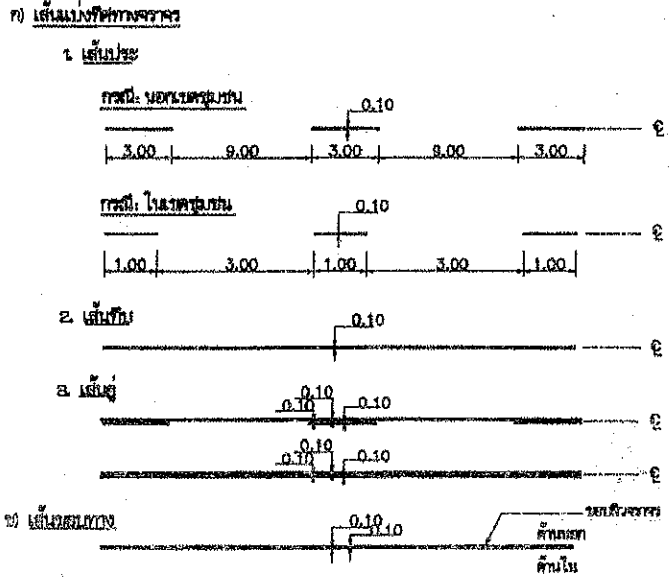
ขนาดและระยะของเครื่องหมายจรรยาบริเวณต่าง
