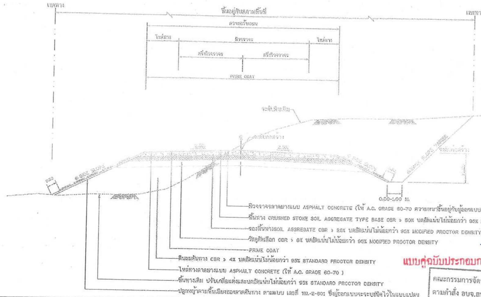
รูปตัดตรงของโครงสร้างถนนดินตัด ดินถมและคลุมสัมนปิดผิว
