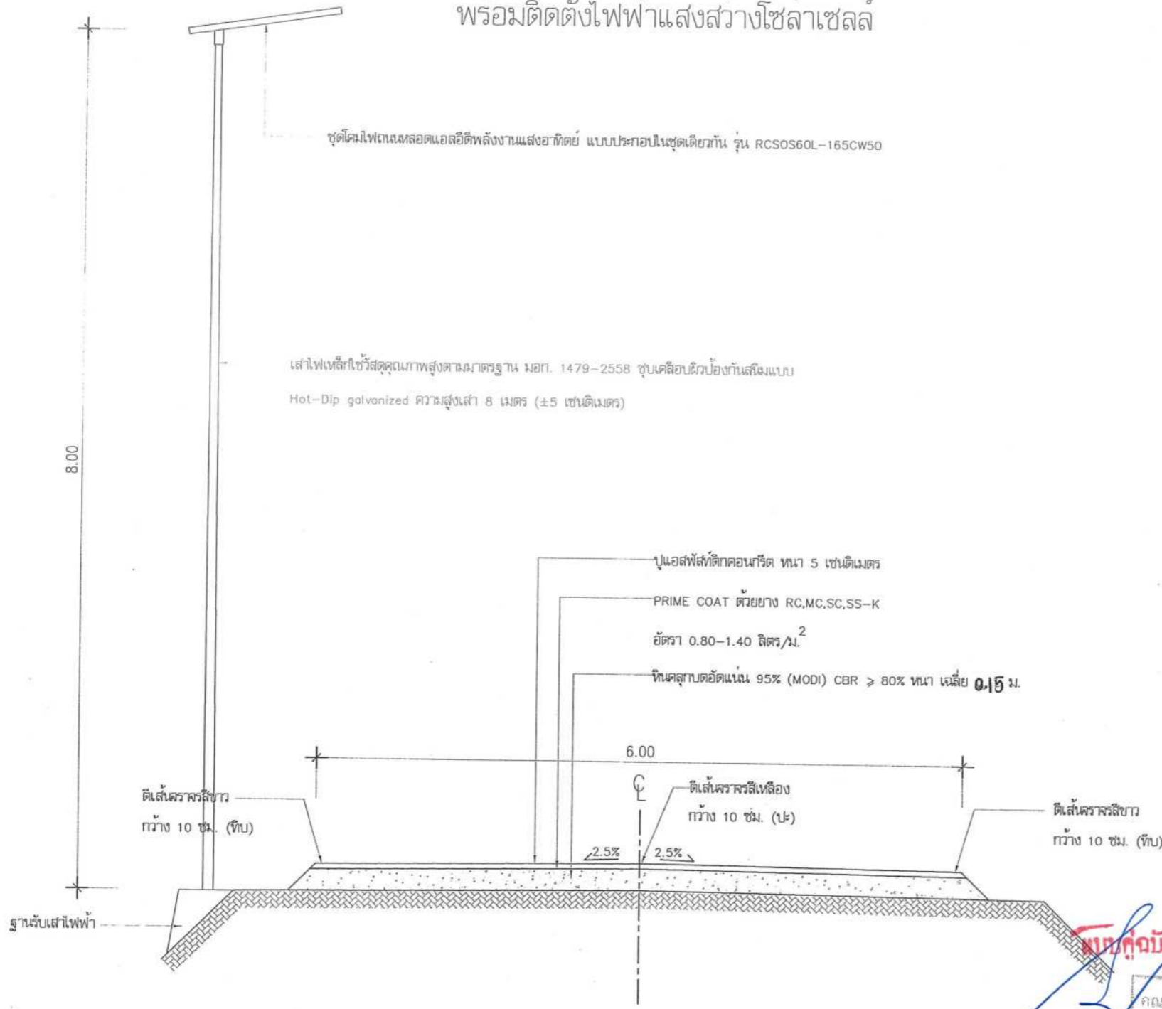
รูปตัดตามขวาง ก่อสร้างถนนลาดยางแบบแอสฟัลต์ติกคอนกรีต (Asphaltic Concrete)
