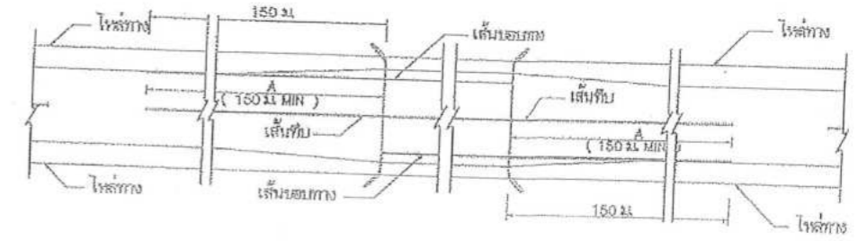
กรณีความกว้างสะพานน้อยกว่าความกว้างจรวดจรดถนน
