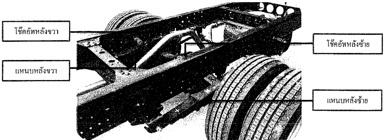
รูปภาพประกอบ ตำแหน่งระบบกันสะเทือนหน้า-หลัง
