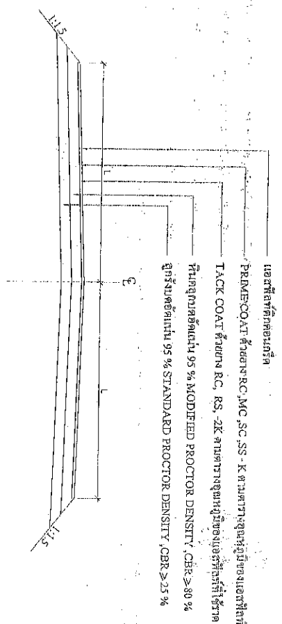
รูปตัดถนน แอสฟัลติก คอนกรีต
