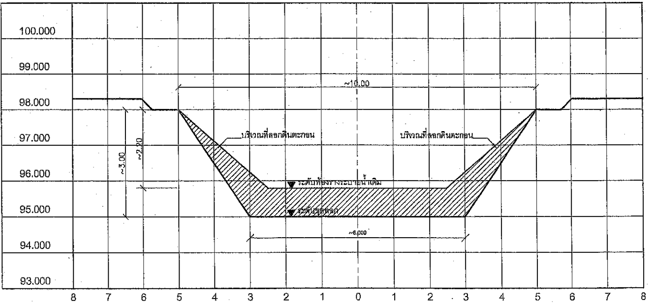
รูปตัดตามขวาง พื้นที่หน้าตัด 7.48 ตารางเมตร
