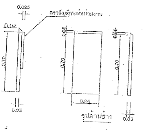
แสดงรายละเอียดแผ่นบุสำเร็จ
