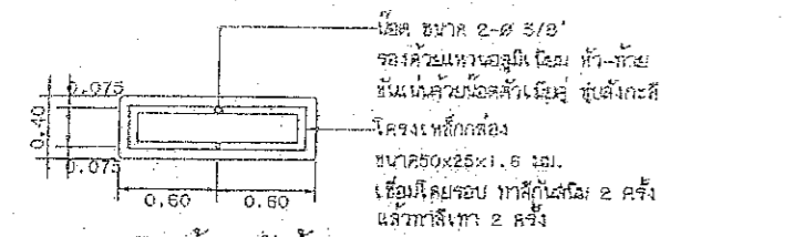
รายละเอียดด้านหลังป้าย N-4
