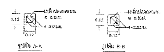
รูปตัดแสดงเสาป้าย
