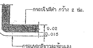
แสดงมุมป้ายแนะนำ (น-2 ถึง น-5)
