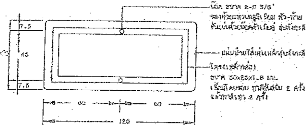
แสดงการยึดโครงป้ายโครงการ N-1
