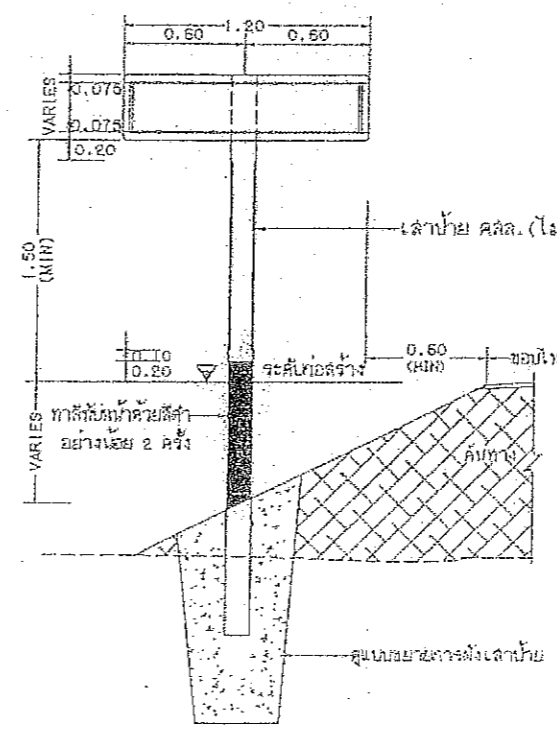
แสดงการปักเสาป้ายแนะนำ N-1 และ N-4
