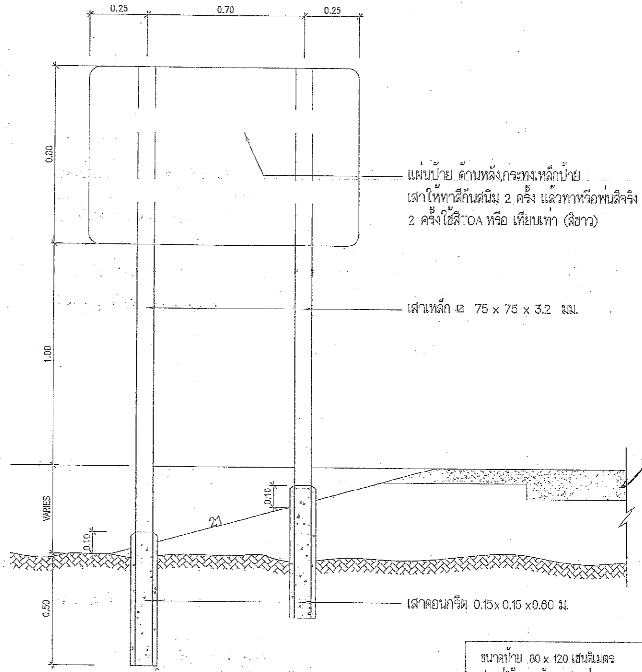
แสดงการปักเสาด้านข้าง
