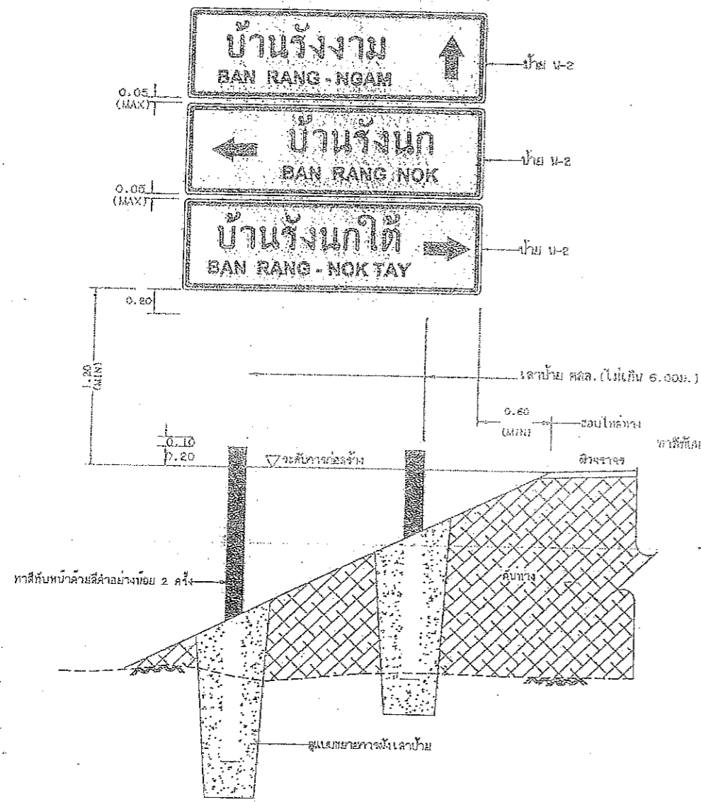
แสดงการติดตั้งเสาป้าย N-2 (ชุด) และ N-3 (ชุด)
