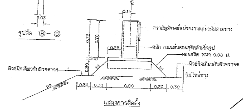
แบบหลักกิโลเมตร แบบที่ 2
