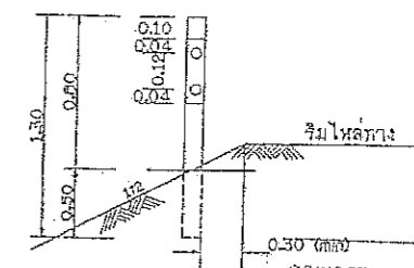
แสดงรายละเอียดการติดตั้งหลักกิโลเมตรแบบที่ 2
