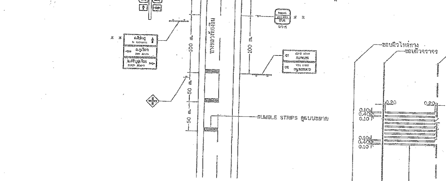
แสดงการติดตั้งป้ายจราจรบริเวณสี่แยก ( เชื่อมทางหลวงท้องถิ่น )
