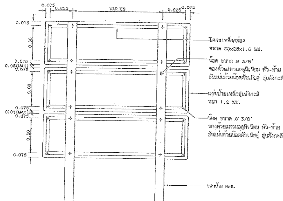
แสดงการยึดโครงเสาป้าย N-2 (ชุด) และ N-3 (ชุด)
