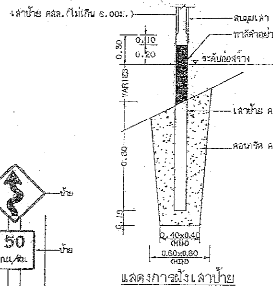
แสดงการปักเสาป้ายแนะนำ N-1 และ N-4
