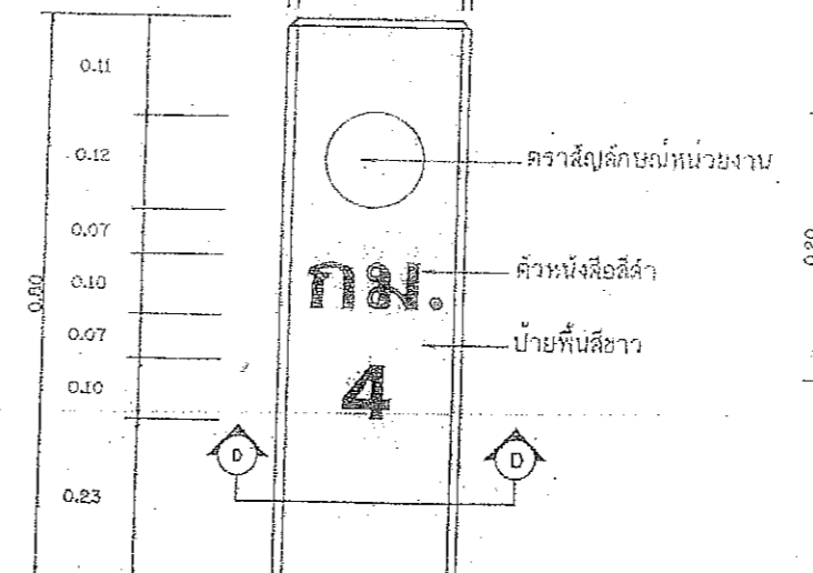
แบบหลักกิโลเมตร แบบที่ 2
