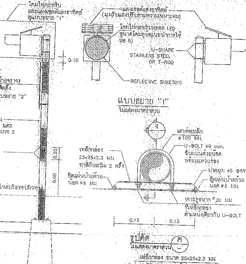
รูปด้านข้าง ไฟกะพริบร่วมกับป้ายจราจร แสดงการติดตั้งสัญญาณไฟกะพริบอย่างเดี่ยวหรือร่วมกับป้ายบังคับหรือป้ายเตือน (เสาเหล็ก) ไม่แสดงขนาดเสา
